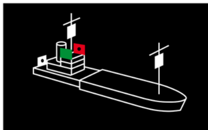
Schubverband in Fahrt (starr verbunden)
