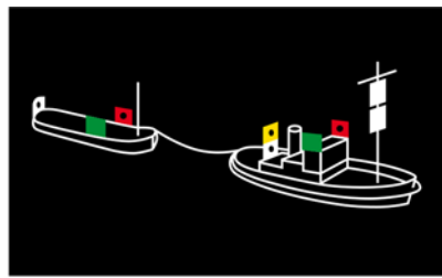
Schleppverbände in Fahrt; bis 200m Schleplänge (Schlepper nicht über 50m Länge)
