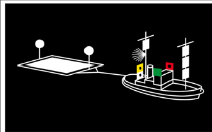
Schleppverbände in Fahrt über 200m Länge, mit außergewöhn- lichem Schwimmkörper (schleppen- des Fahrzeug über 50m lang)
