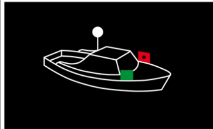
Maschinenfahrzeug in Fahrt unter 7 m Länge, 7 kn Höchstgeschwindigkeit
