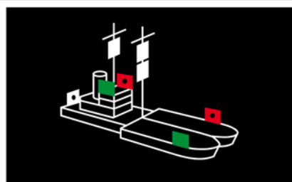
Schubverband in Fahrt (nicht starr verbunden) schiebendes Fahrzeug über 50m lang
