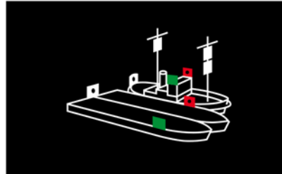
Schleppverbände in Fahrt; bis 200m Schleplänge mit längsseits geschleppten An- hängen
