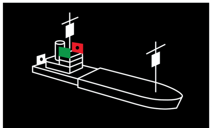
Schubverband in Fahrt (starr verbunden)
