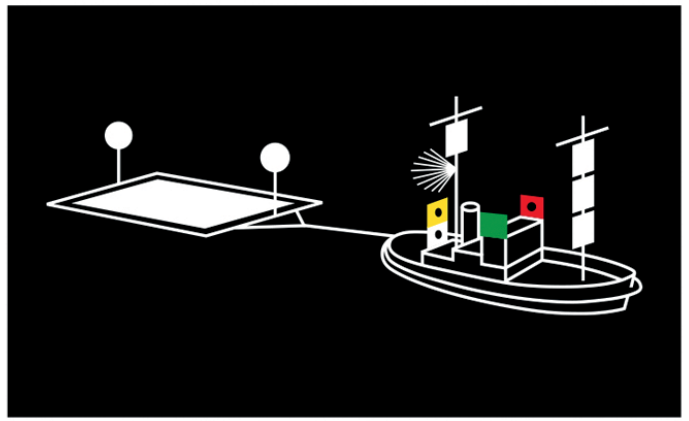
Schleppverbände in Fahrt über 200m Länge, mit außergewöhnlichem Schwimmkörper (schleppendes Fahrzeug über 50m lang)
