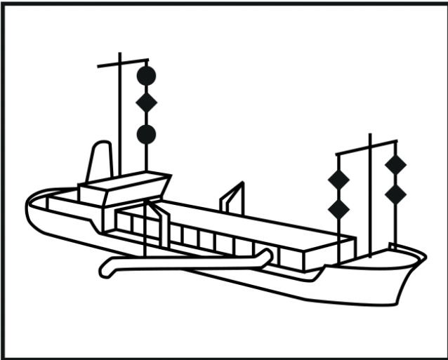
Manövrierbehindertes Fahrzeug bei Bagger- oder Unterwasserarbeiten
