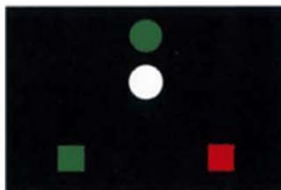
Frei fahrende Fähre
